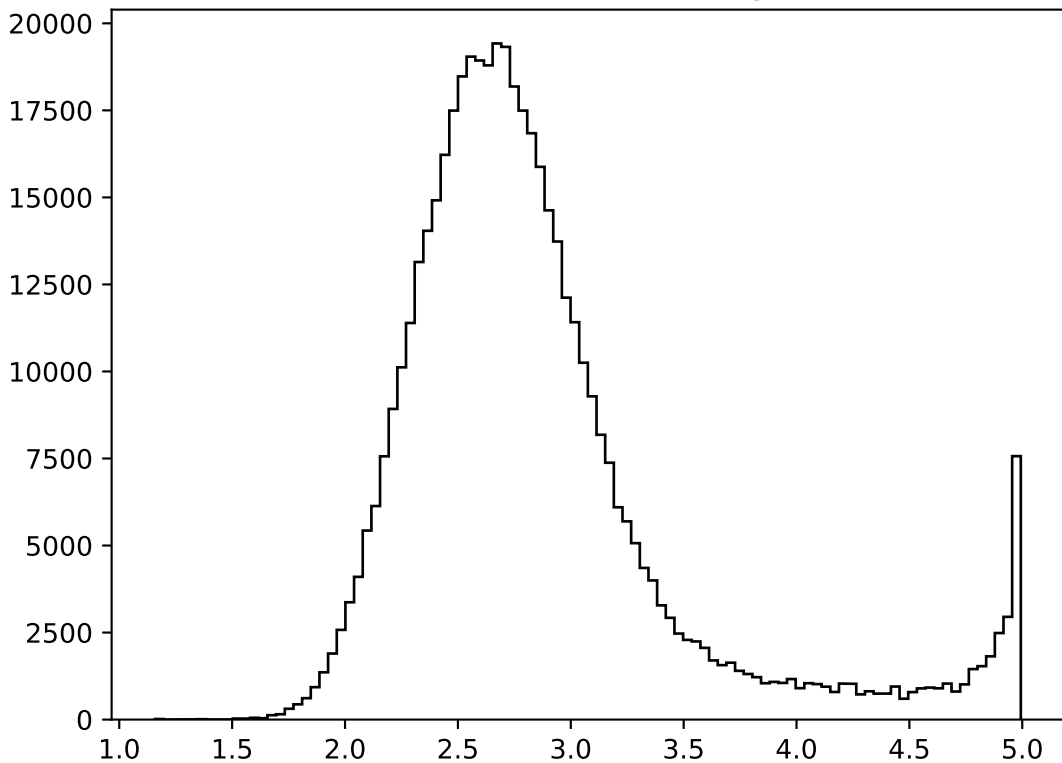
ColourReconnection:range=
