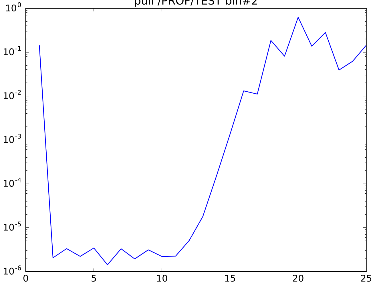
pull /PROF/TEST bin#2
