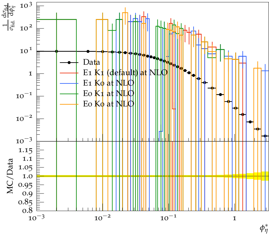
\phi_\eta^* spectrum, Z \rightarrow e\bar{e} (bare)
